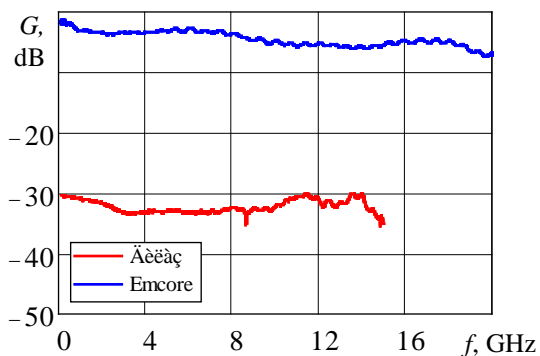
Рис. 5. АЧХ линий Дилаз и Emcore
