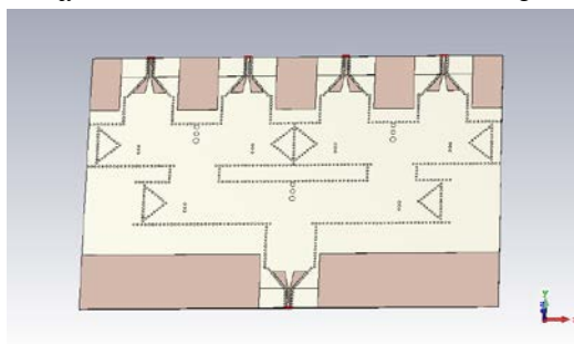
Рис.4. Делители/сумматоры мощности
