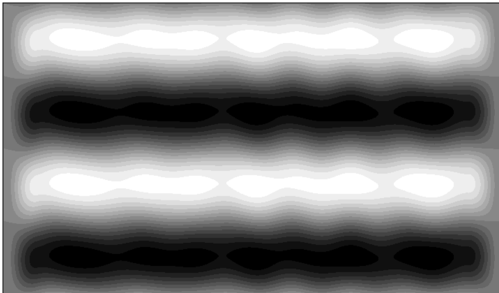
Рис. 2. Развертка амплитуды деформации поверхности волноводного преобразователя.
