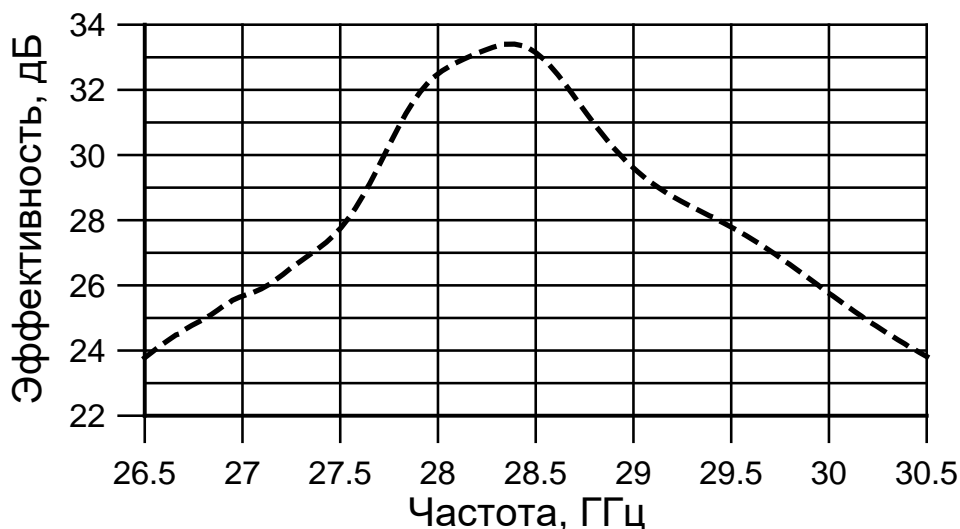
Рис. 3. Эффективность поляризатора в зависимости от частоты.
