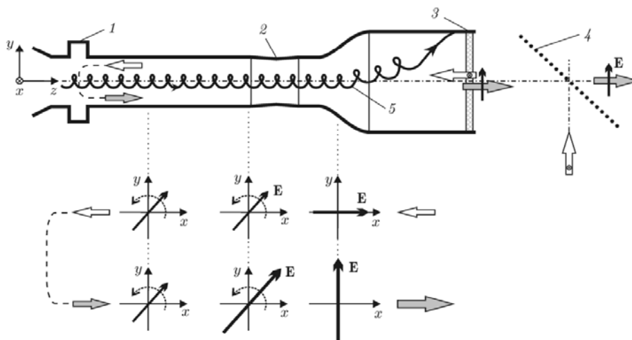
Рис. 1. Схема ввода и вывода излучения gyro-ЛБВ через одно окно. 1 – отражатель, 2 – поляризатор, 3 – окно, 4 – сплиттер.
