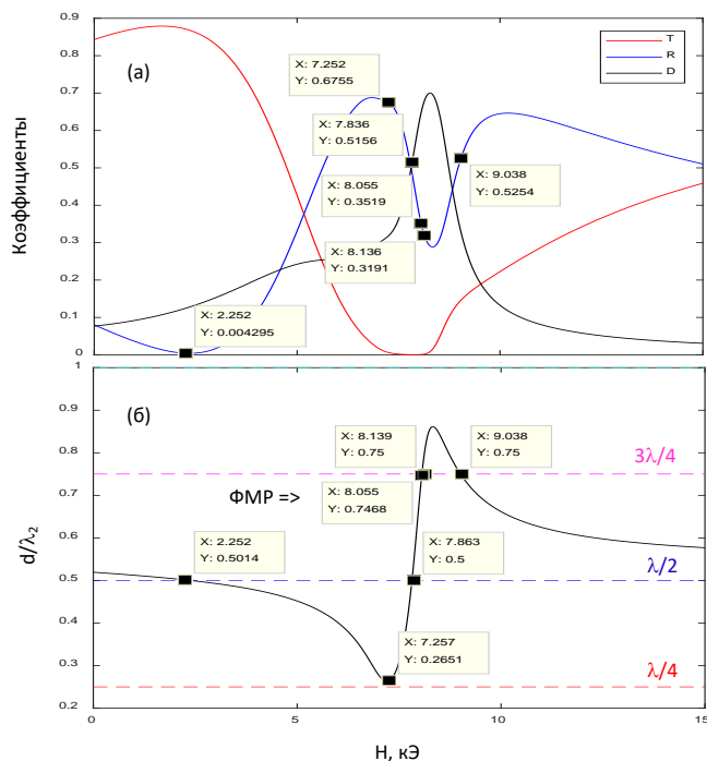
Рис. 3. Идентификация резонансов в пластине ЖИГ (образец №2) на полевых зависимостях коэффициентов – (а) и отношения толщина пластины/длина волны – (б).
