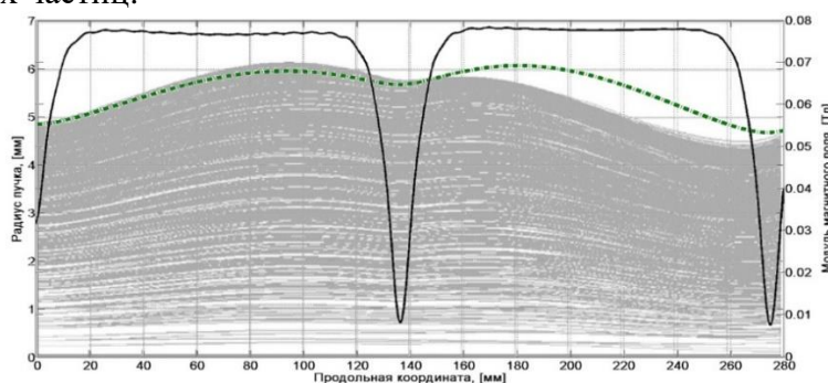
Рисунок 2. Траектории пучка в РМФС, полученные численным моделированием и контур пучка, рассчитанный по уравнению (3).
